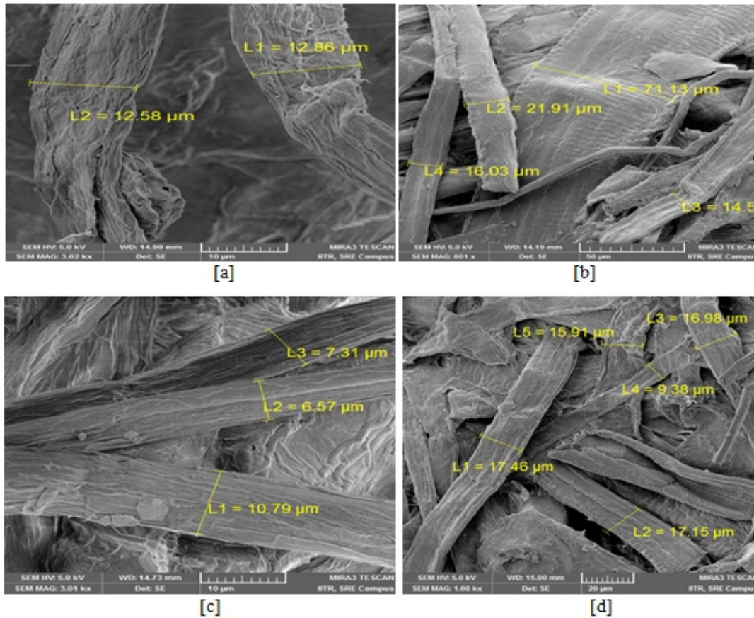
Fig. 12 FE-SEM micrographs of [a] KC, [b] KA, [c] SC, [d] SA
